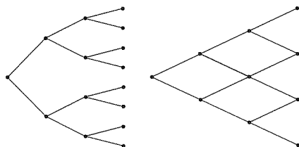
(a) Binomial tree
